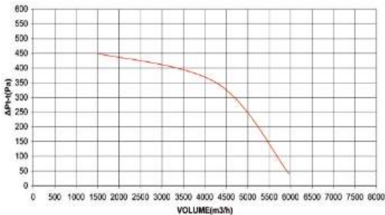
Ø250-1.5HP-1450RPM
